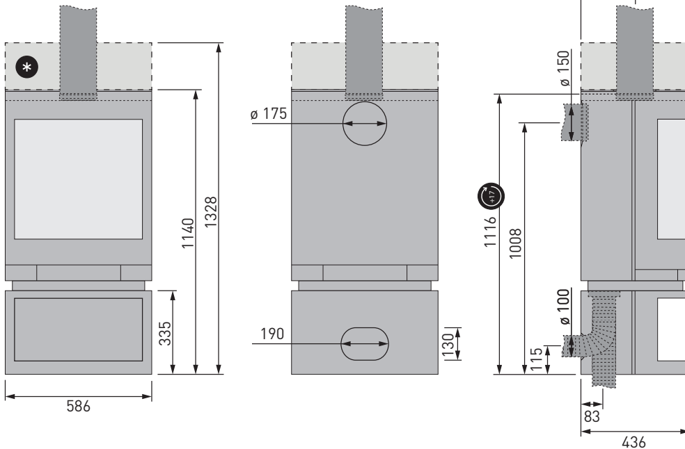
Vista frontale
