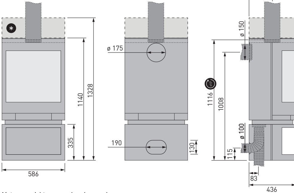
Voorraanzicht
