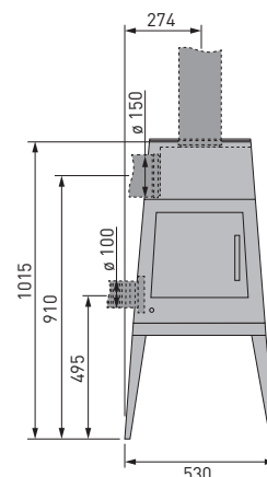
Vista laterale
