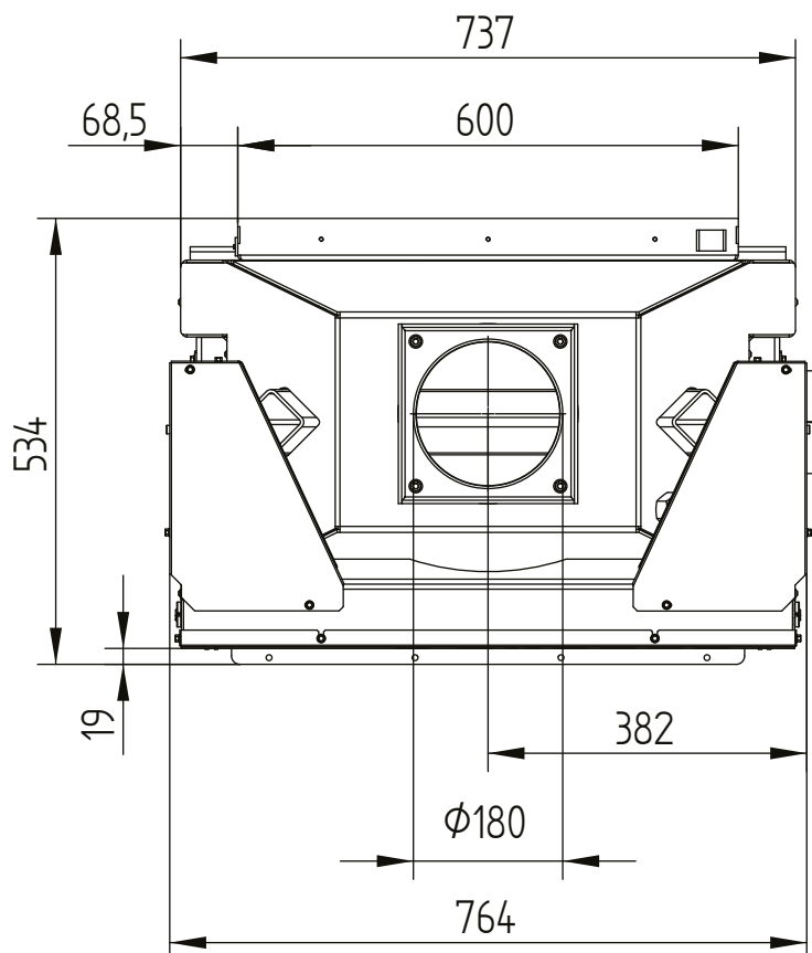
Hochschiebbare Tür
